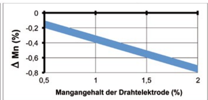
Ab-/Zubrand von Mangan
