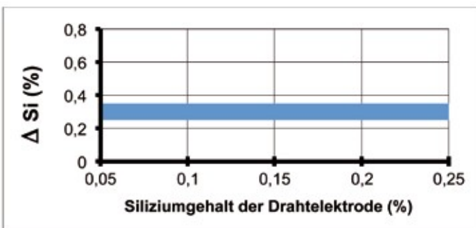
Zubrand von Silizium
